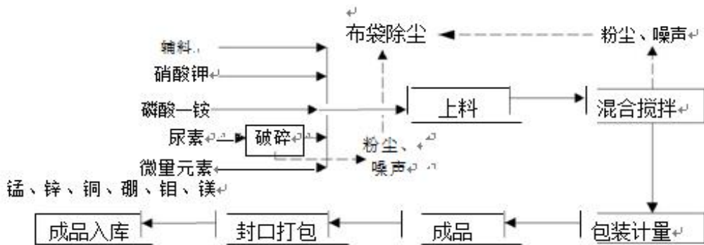
图 2-3 固体水溶肥工艺流程及产污环节图
