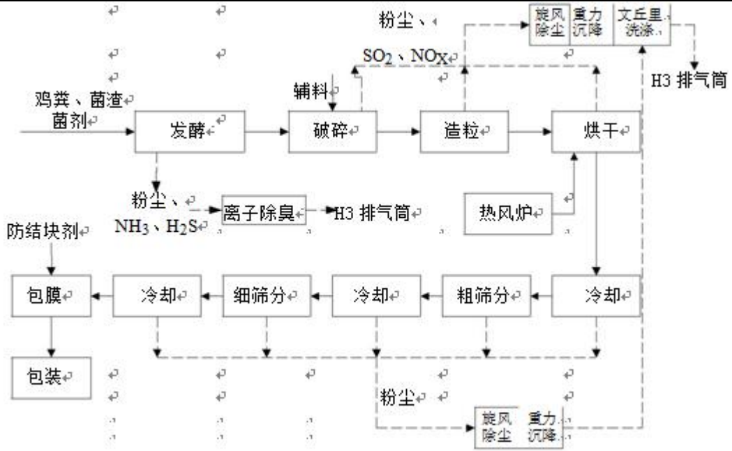
图 2-5 有机肥工艺流程及产污环节图
