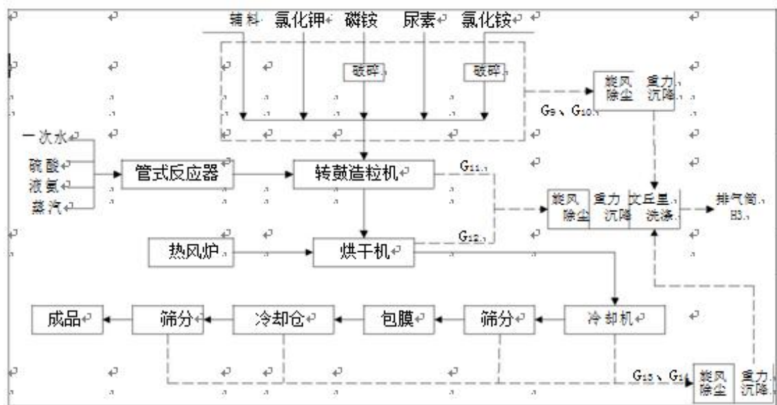
图 2-1 氨酸缓释复合肥工艺流程及产污环节图
