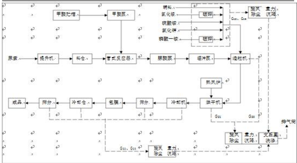
图 2-2 氨脲缓释复合肥工艺流程及产污环节图
