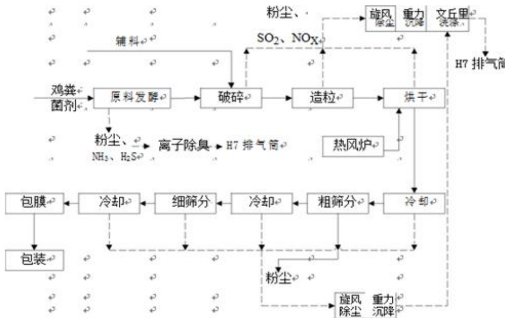
图 2-6 生物有机肥工艺流程及产污环节图
