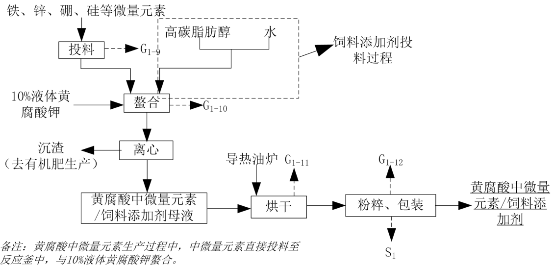
图2-7 黄腐酸中微量元素/饲料添加剂项目生产工艺流程及产污环节图
