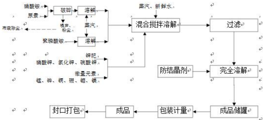
图 2-4 液体水溶肥工艺流程及产污环节图
