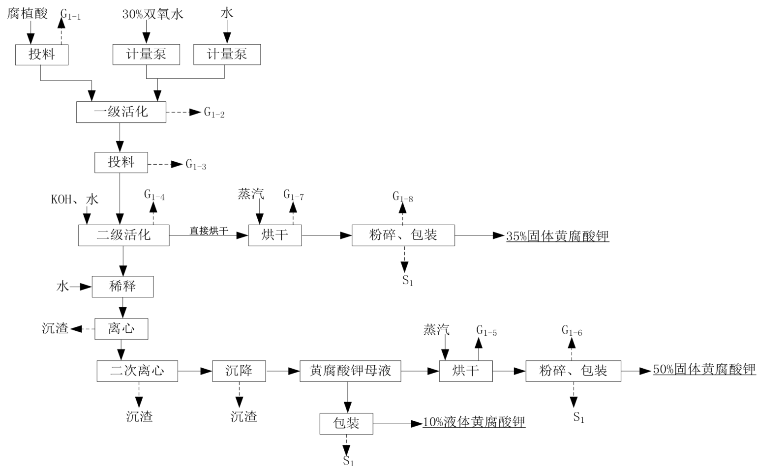
图 2-8 黄腐酸钾原液、原粉生产工艺流程及产污环节图
