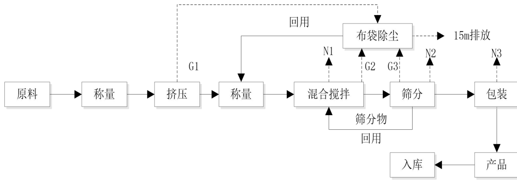
图 2-9 掺混肥生产线生产工艺流程图及产排污环节
